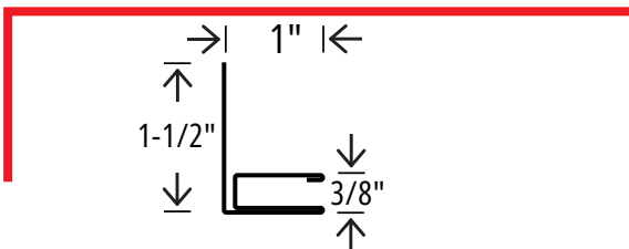
Mitre Divider Moulding (Aluminum)
