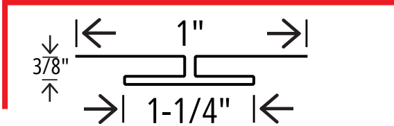
Mitre Divider Moulding (Aluminum)
